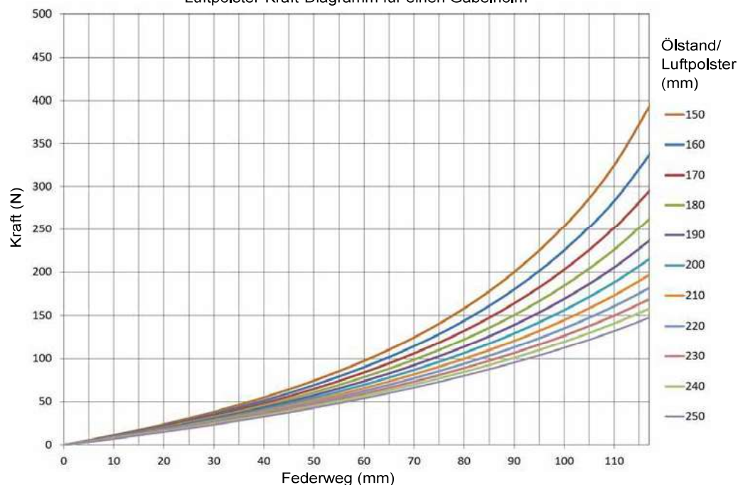
Luftpolster-Kraft-Diagramm für einen Gabelholm
